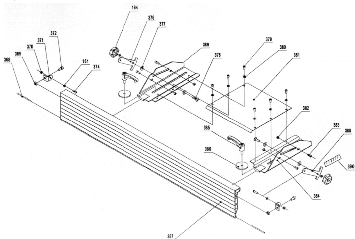
Рисунок 31. Параллельный упор
